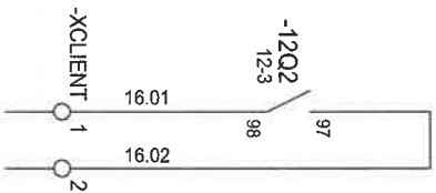
DISJONCTION PPE-M1
