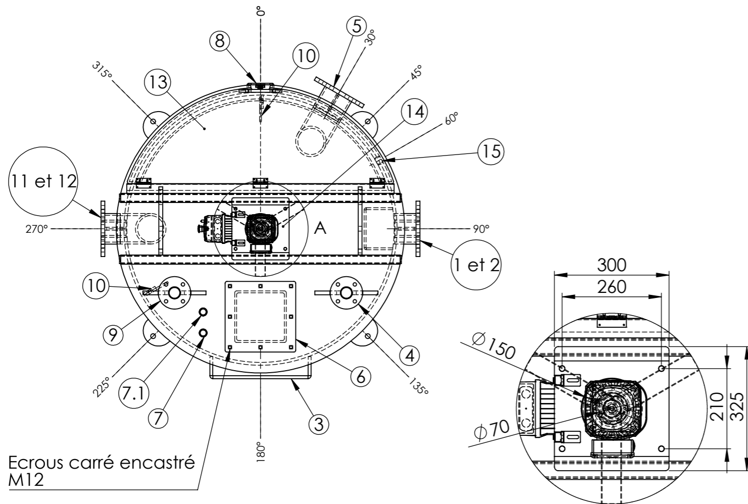
DÉTAIL A ECHELLE 1 : 10
